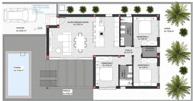
VIVIENDA TIPO 'B' 1:100
